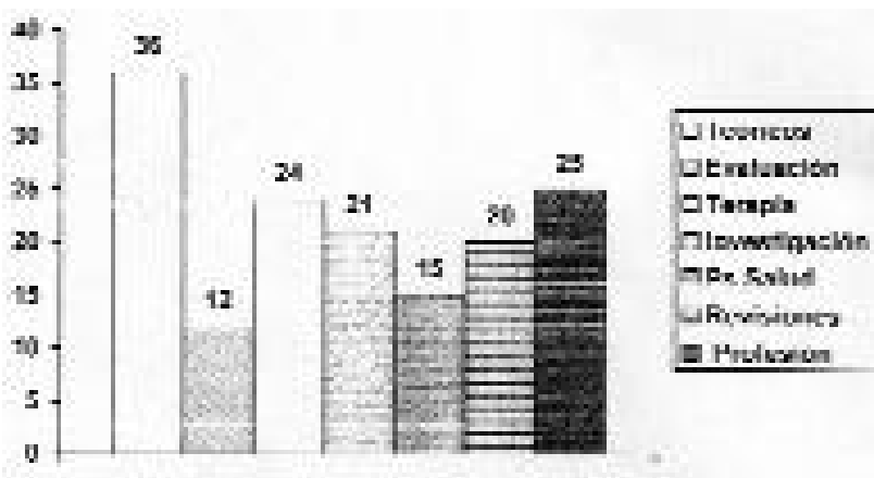
FIGURA 2 Categorías temáticas
