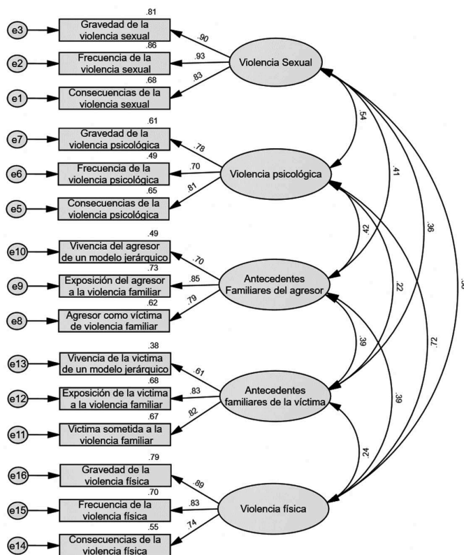
Figura 1. Diagrama de ruta del modelo reespecificado para el análisis factorial confirmatorio.
